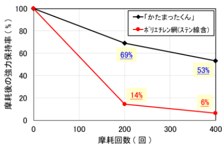
摩耗試験後の強度保持率
